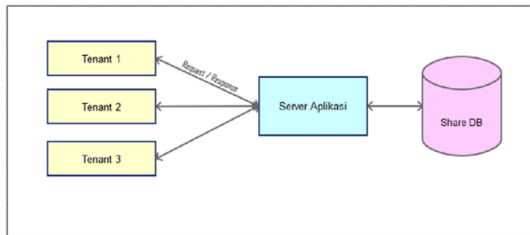
Gambar 2. Arsitektur Multitenancy Basis Data Berbagi
