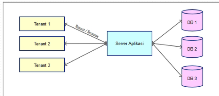
Gambar 1. Arsitektur Multitenancy Basis Data Terpisah
